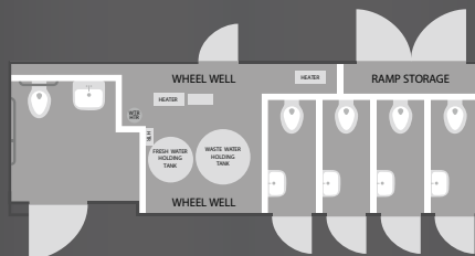
8x26' ADA PLUS 4 FLOOR PLAN
